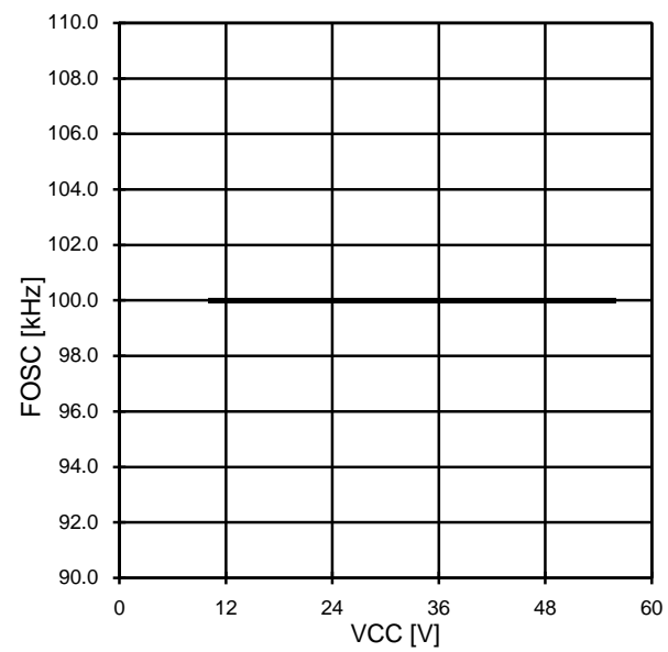
Fig.2 FOSC-VCC
