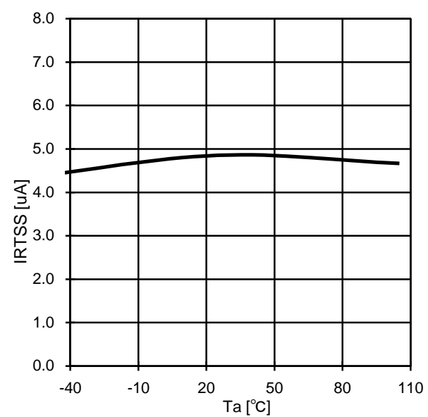
Fig.4 IRTSS-Ta (VRTSS=1V)
