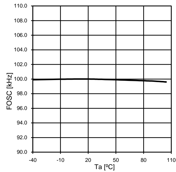
Fig.1 FOSC-Ta
