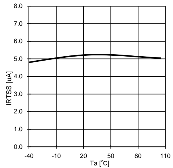
Fig.3 IRTSS-Ta (VRTSS=0V)
